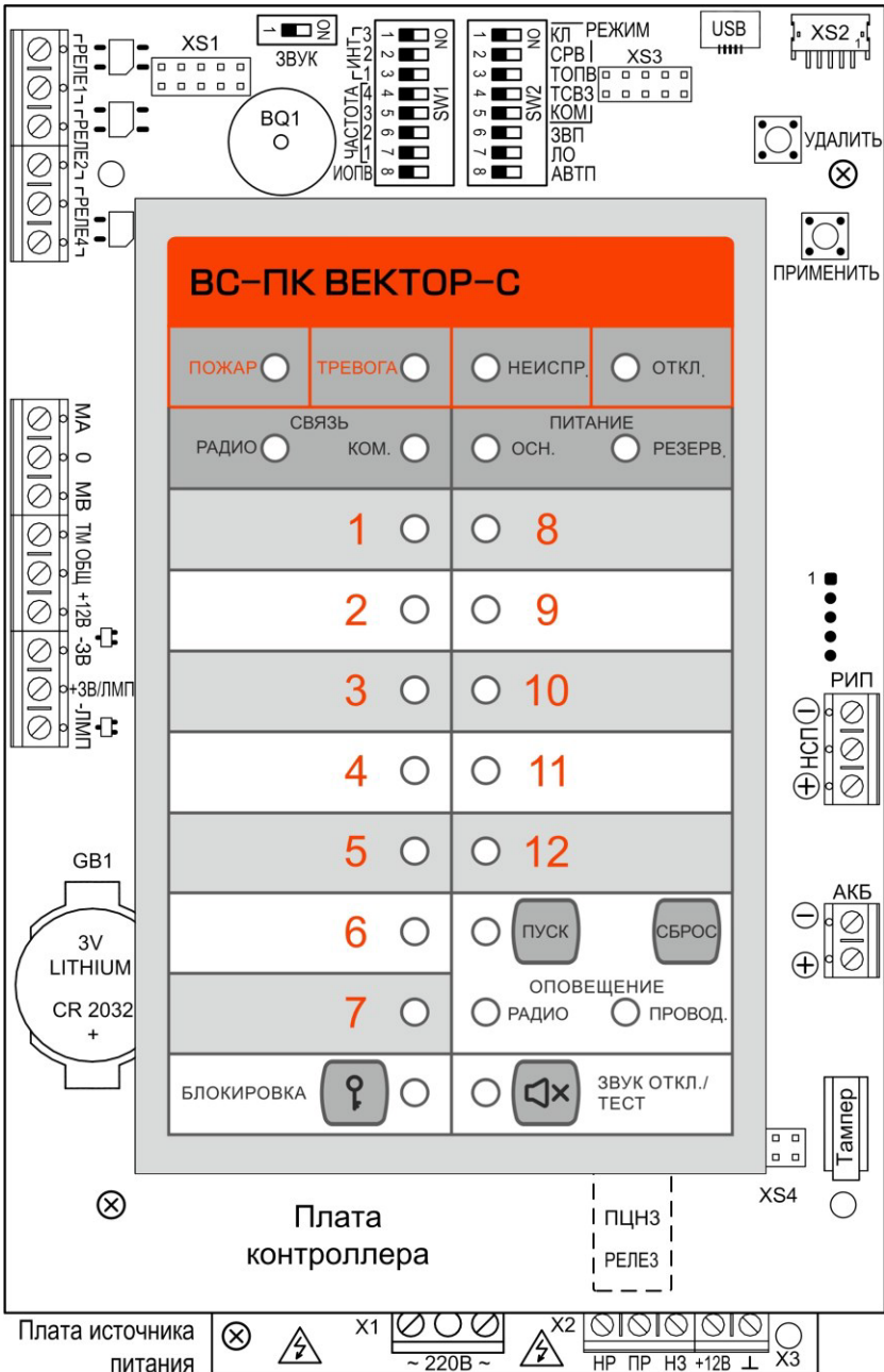
Рис.А1. Плата прибора «ВС-ПК ВЕКТОР-С SN»
