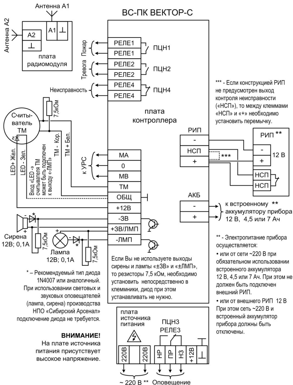
Рис.А2. Схема внешних соединений прибора «ВС-ПК ВЕКТОР-С SN»
