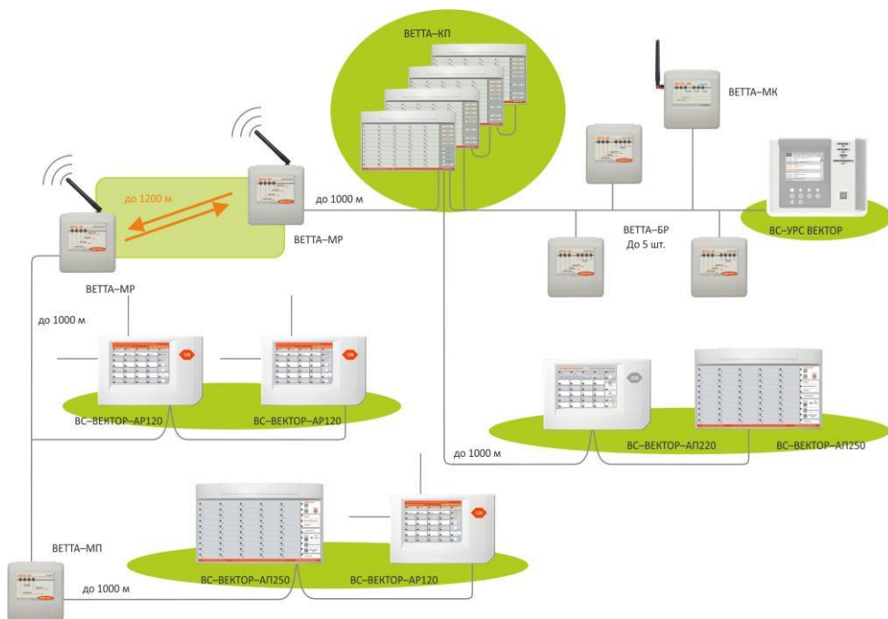
Рис. 2 Пультовая система, система передачи извещений «БЕТТА – 2020»
